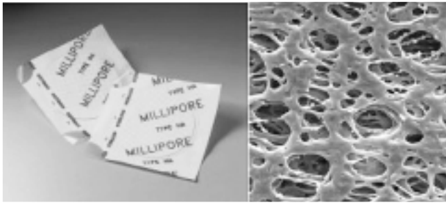
Figura 5-19: FILTRO DE ACETATO DE CELULOSA “MILIPORE” VISTO AL MICROSCOPIO
